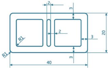
LEGAR 20 X 40 MM
