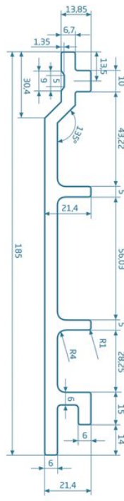
PROFIL ELEWACYJNY 185 X 21,4 MM
