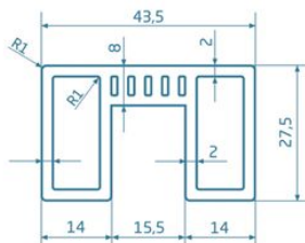
LISTWA OGRODZENIOWA C 1750 X 27,5 X 43,5 MM
